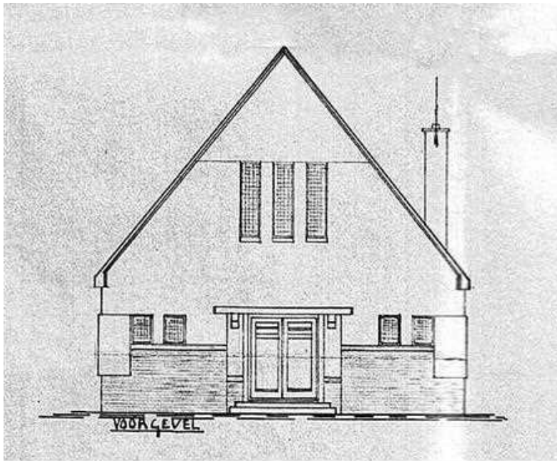
De bouwtekening uit 1933 Collectie oud archief Gemeente Lichtenvoorde
