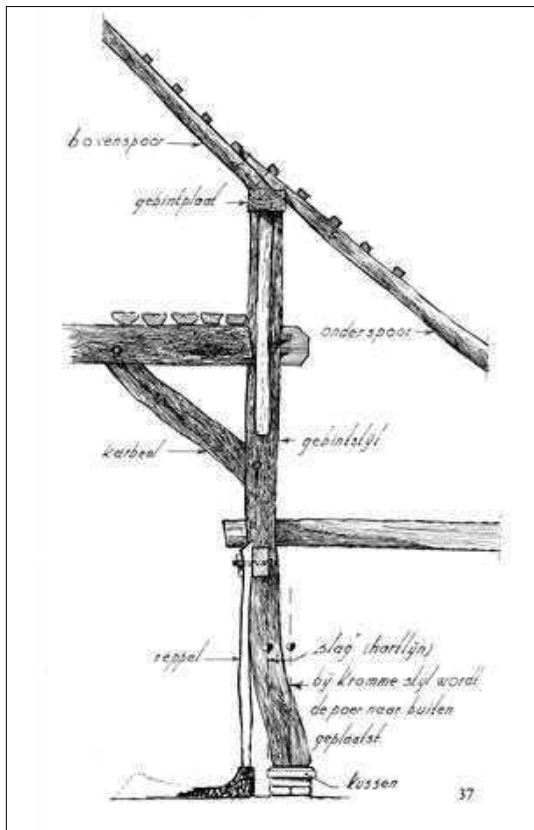
Gebintwerk zoals dat vroeger bij de bouw van boerderijen werd toegepast. Tekening uit boek: De vakleu en et vak van L.A. van Prooije
