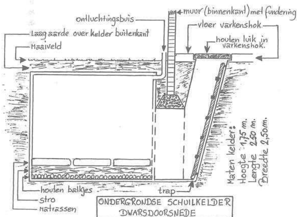
Dwarsdoorsnede van de ondergrondse schuilkelder.
