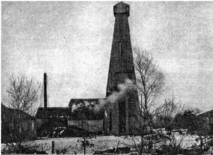
De aardolievondst te Corle bij Winterswijk. Het is te hopen, dat men hier inderdaad een winstgevende bron van petroleum heeft gevonden, die in de toekomst van groot belang voor ons Land zal zijn. Bovenstaande foto brengt den boortoren in beeld.
